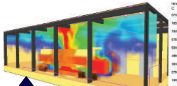
Yangın kompartımanında ısı yayılım analizi
