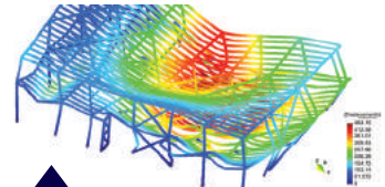
Yangın anında çelik konstrüksiyonun davranışı ve hasar analizi
