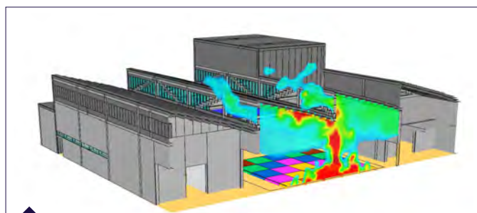
Propagation des fumées dans un grand volume (hall)
