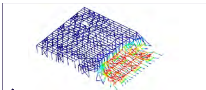
Simulation du mode de ruine d'une structure (ICPE)
