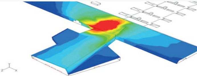
Tren istasyonu döşemesinde sıcaklık dağılımı
