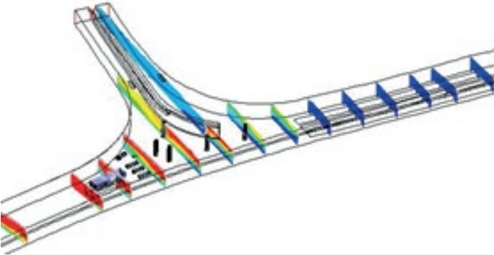
Tünel içerisindeki bir araç yangınının CFD analizi
